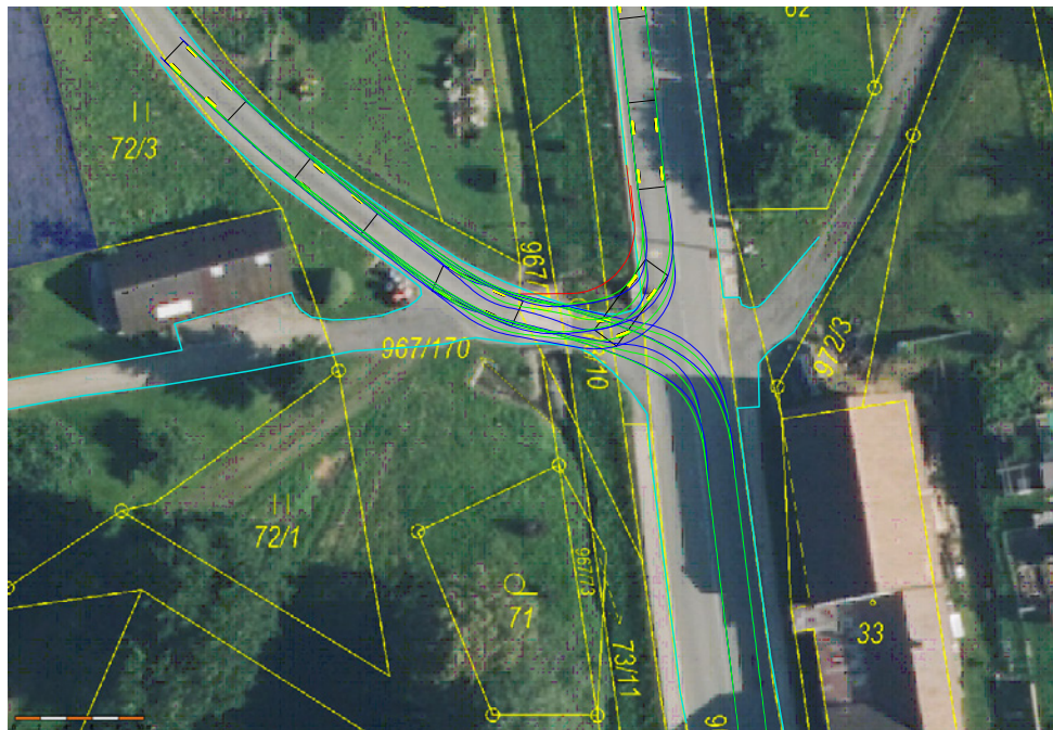
SITUACE FORD TRANSIT DLOUHÝ
